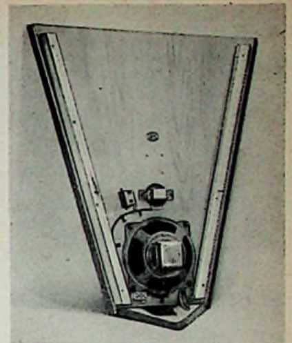
Bild 11. Cophon-Schallecke, Rückansicht einer Eckenlautsprecherkombination von Lorenz
