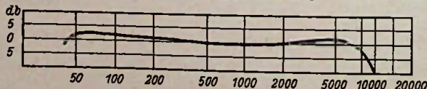
Bild 1. Frequenzkurve des Bändchenmikrofons M 31 von Beyer
