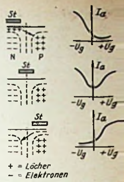
Bild 5. Einfluß der Stellung der Steuerelektrode auf den Anodenstrom eines p-n-Fieldistors
