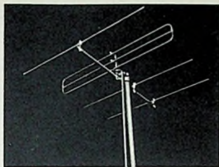
UKW-Horizontal-Rahmen-Antenne
