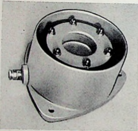
Bild 6. Schußgeschützter Lautsprecher für rauhesten Betrieb auf Schiffen (Ultraton)
