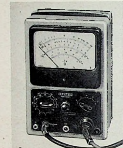
Grundig-Universal-Röhrenvoltmeter
