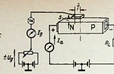
Bild 4. p-n-Fieldistor
