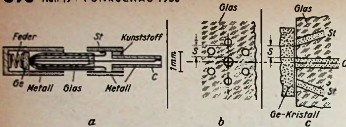
Bild 3. Punktcontact-Fieldistor. a = Schnitt durch die Anordnung, b = Aufsicht auf die Elektroden, c = Schnitt durch die Elektroden
